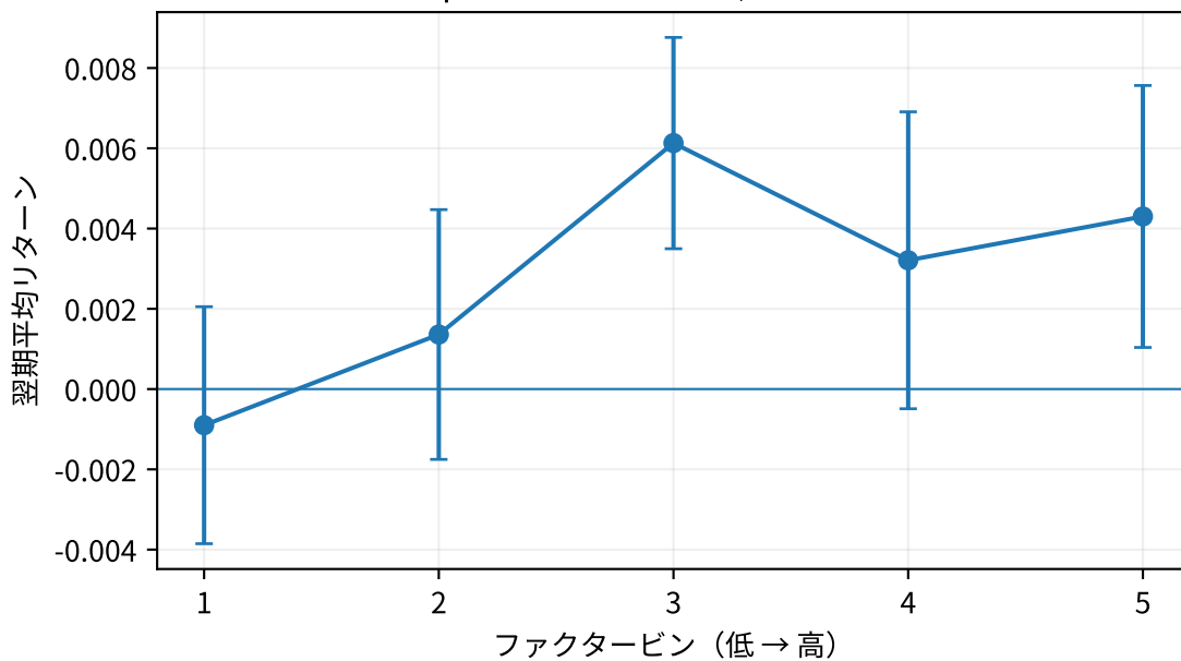
FA1001 12か月モメンタム Top-Bottom=0.440%, 単調性=0.75
